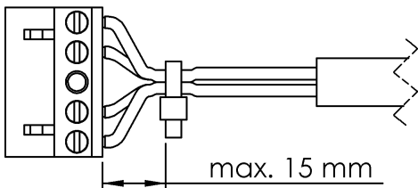
Klemme Netzanschluss
