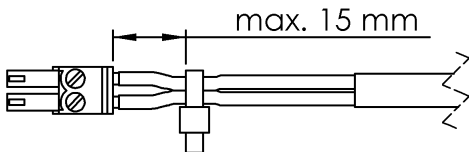
Klemme Fühleranschluss
